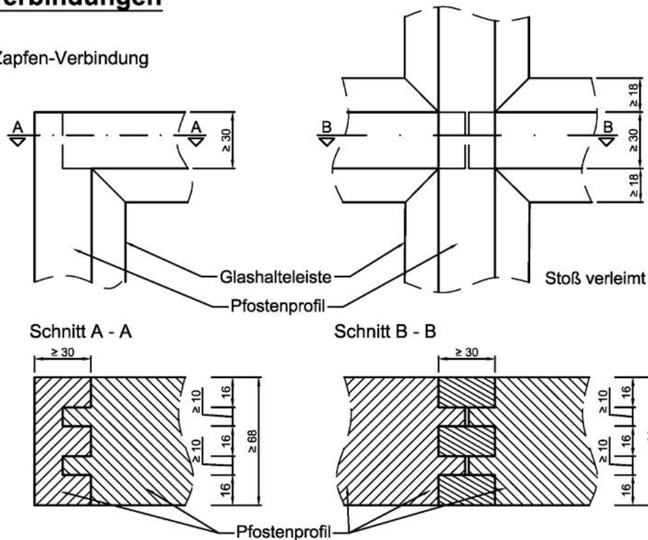
wahlweise Flachdübel-Verbindung
